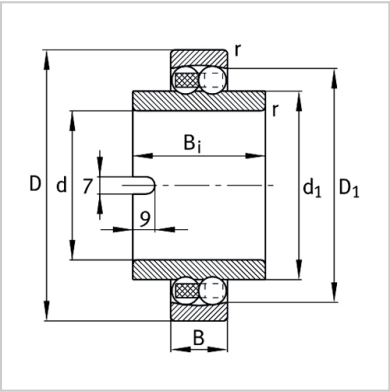
加宽内圈
