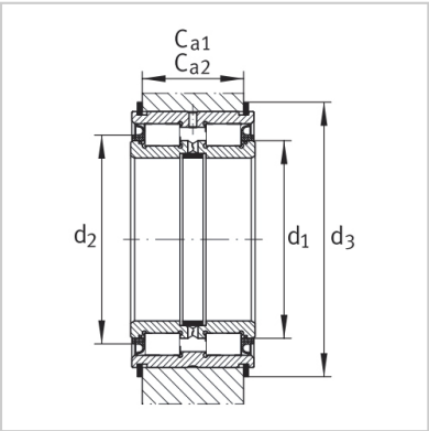
安装尺寸
